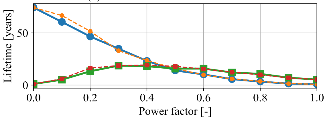
(d) IGBT and diode estimated lifetime
